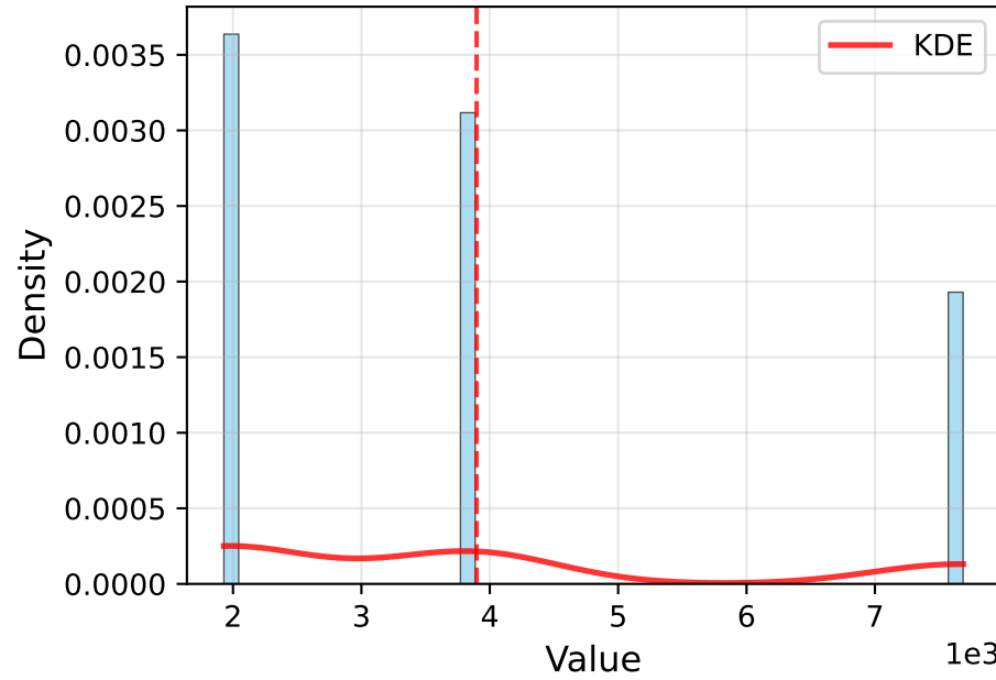
Input Tokens \mu=3897.40 , \sigma=2179.75
